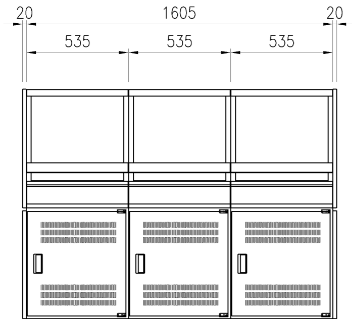
3bay
