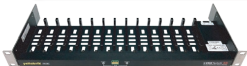
RFR 1000-1 19 インチ 1U ラックフレーム yellobrik 14 台まで搭載可能。別売りの電源アダプタ (RPS1120) プライマリ用とリダンダント用の 2 つを接続可能。 (yellobrik14 台に電源一括供給)
